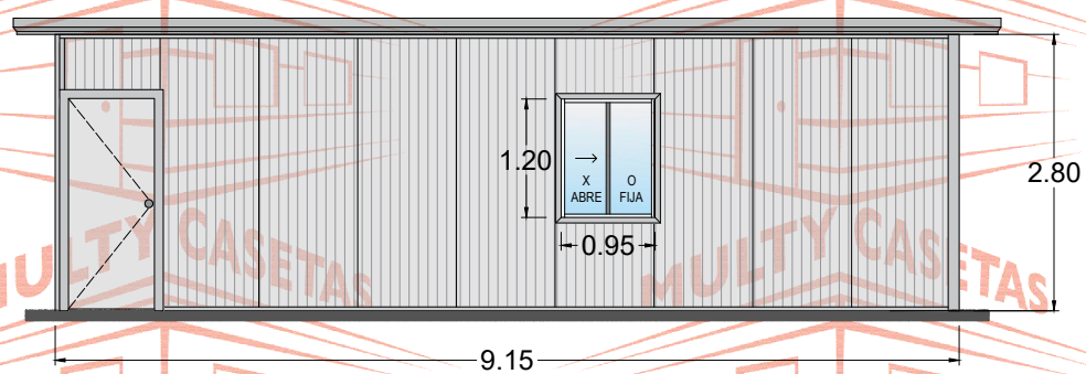
FACHADA FRONTAL
